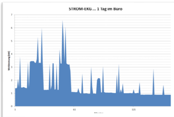
Abbildung 1 – Beispiel Lastgang Bürotag
